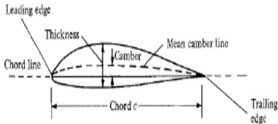
FIG 6 : Airfoil Nomenclature
